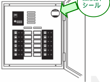
分電盤
