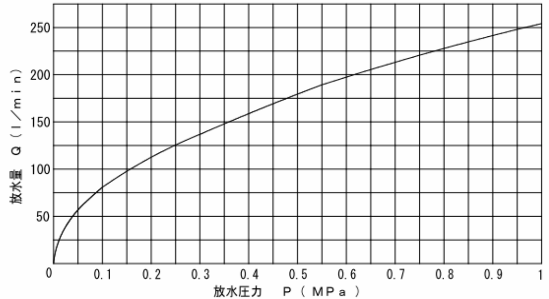
圧力-放水量曲線 流量定数 K=80 (Q=K\sqrt{10P})
