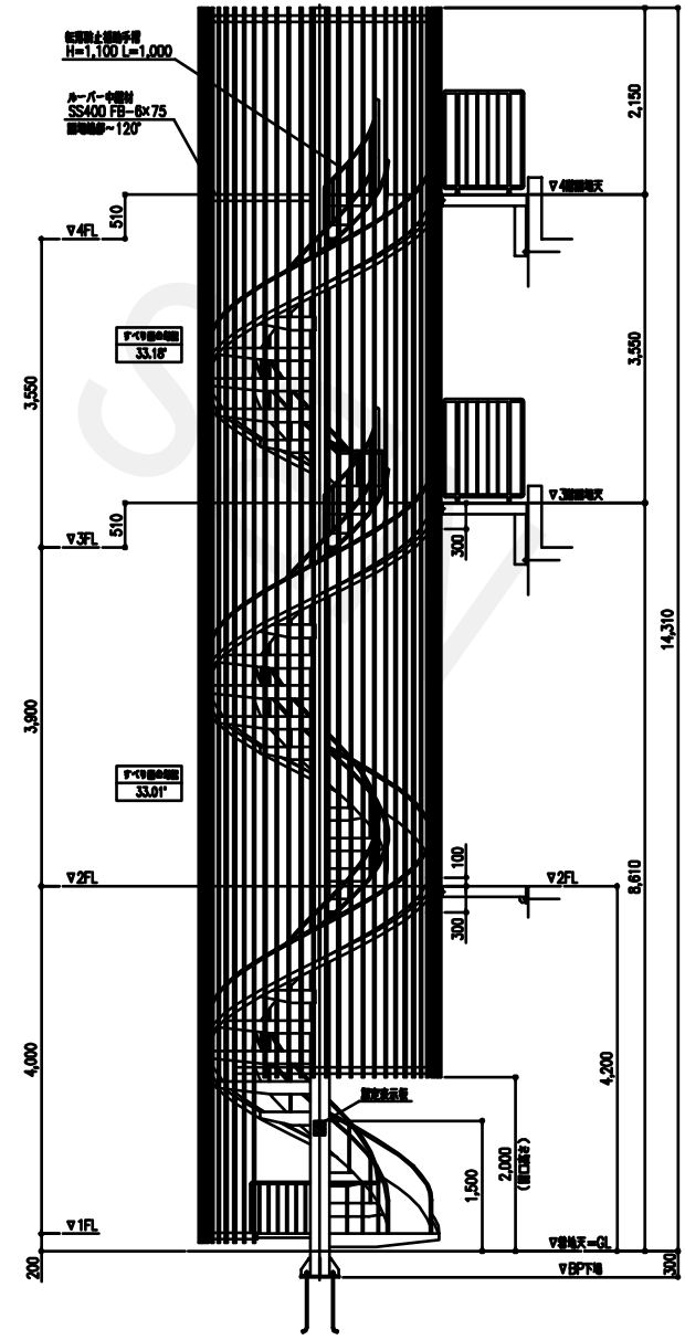
立面図 1:40
