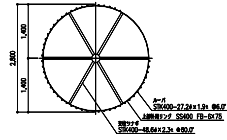
ルーパー天平面図 1:40
